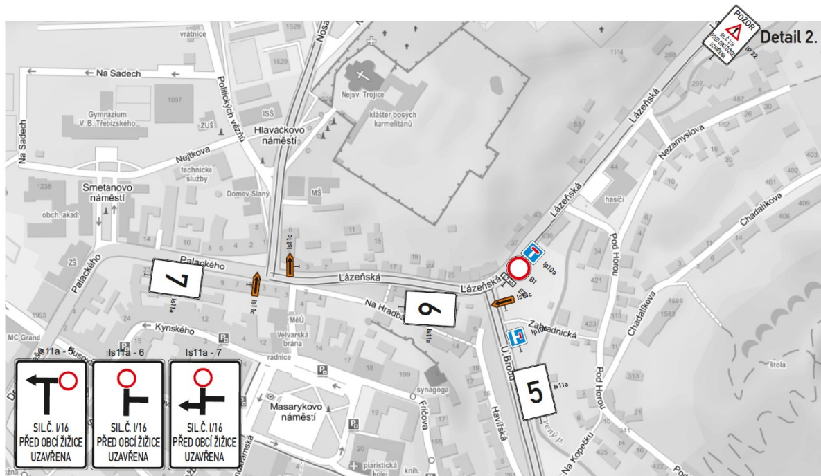
Přechodné dopravní značení – silnice I/16 Lázeňská, Slaný
