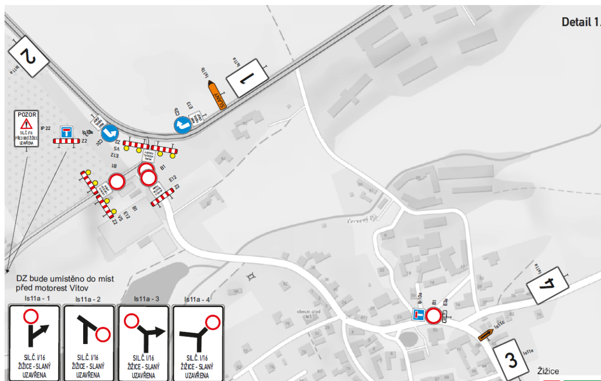
Přechodné dopravní značení – křižovatka silnic I/16 a I/16J
